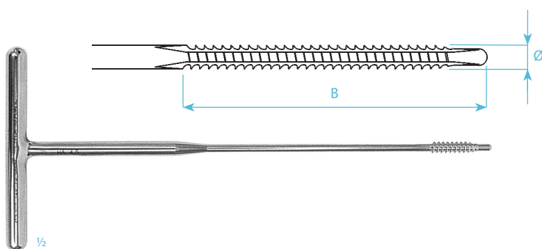
Závitník kortikální Cortical tap
