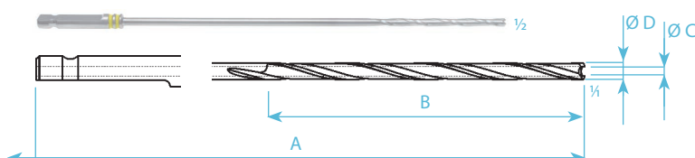
Vrták kanylovaný – koncovka s ploškou Cannulated drill – flat connection
